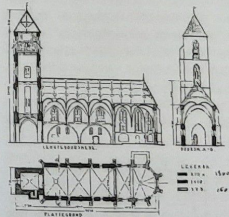
Plattegrond en doorsneden N. H. kerk te Havelte, n. opn. van arch. H. M. Hulsbergen.
